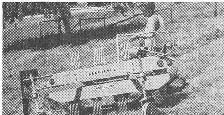
Faneuse de montagne «Heuwiesel»
