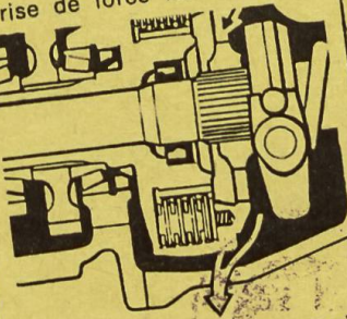
Embrayage turbohydraulique
