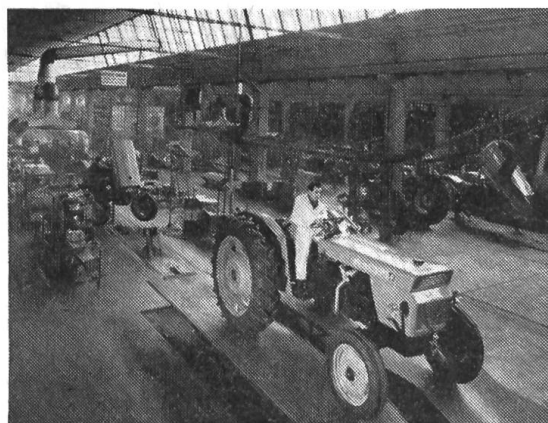
Fig. 2: Les tracteurs «Centauro» quittent les chaînes de montage des Ets SAME de Treviglio à des intervalles de quelques peu de minutes.
