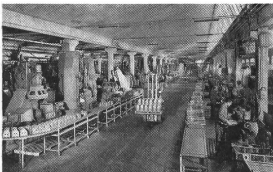
Fig. 1: Vue intérieure partielle des établissements SAME. On voit au premier plan les machines «transfert», projetées et construites la plupart par l'usine SAME elle-même.
