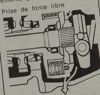
Embrayage turbohydraulique
