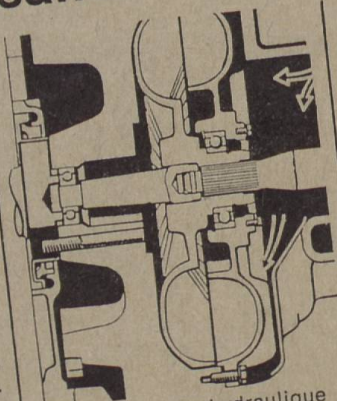
Embrayage turbohydraulique
