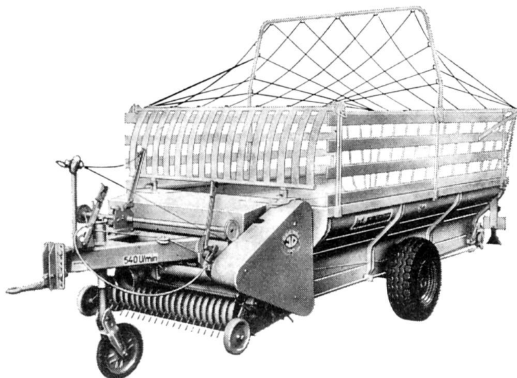
Voici l'auto-chargeuse LELY-DECHENTREITER, modèle LW 2 K
