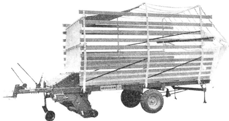
Autochargeuse HAGEDORN «LD»
