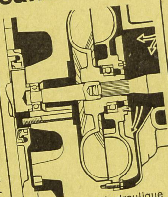
Embrayage turbohydraulique
