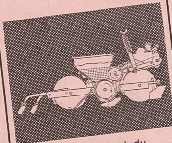
Coupe d'un agrégat du semoir
