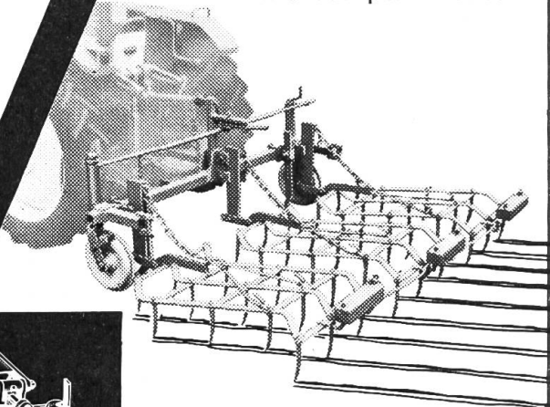
châssis avec herse à 3 compartiments
