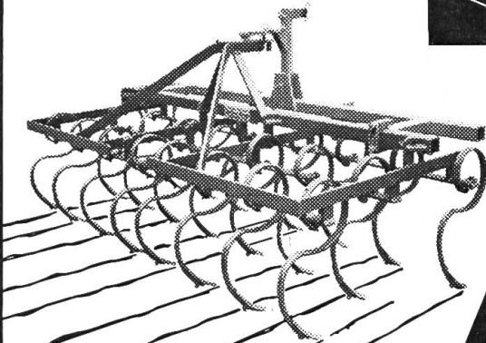
châssis avec cultivateur à dents flexibles
