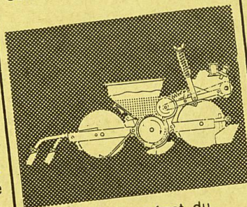
Coupe d'un agrégat du semoir
