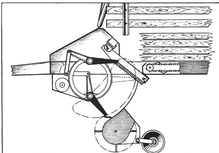
Fonctionnement du mécanisme oscillant double à l'autochargeuse type LD avec dispositif de coupe (coupe à la manière de ciseaux).
