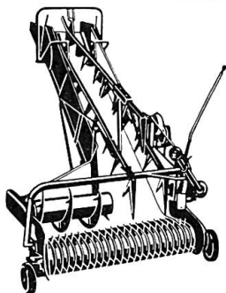
Ramasseuse-chargeuse SL 160 avec ruban expulseur pour le chargement du foin des fourrages verts, du maïs, etc. Largeur de ramassage 1,60 m. Hauteur de charge 3,30 m.
