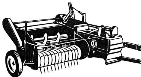
Presse ramasseuse à haute densité Type 214T + Type CB 300 pour le foin et la paille. Largeur de ramassage 1,60 m. Rendement horaire : paille 7 tonnes, foin 9 tonnes.
