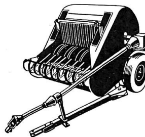
Presse ramasseuse F 81 pour le pressage et le chargement du foin et de la paille. Largeur de ramassage 1,40 m. Rendement horaire 4 à 8 tonnes. Livrabale avec élévateur pour le fourrage vert.
