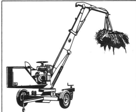
CERES, la grue à fumier hydraulique, exécution à deux roues. Facile à manœuvrer. Service simple.
