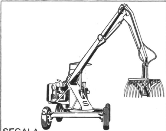
SEGALA, la grue à fumier sur quatre roues. Grande puissance d'élévation. Manipulation simple. Construction robuste.
