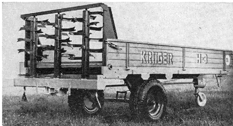
Modèle H-3, l'épanduse de fumier la plus vendue en Suisse
