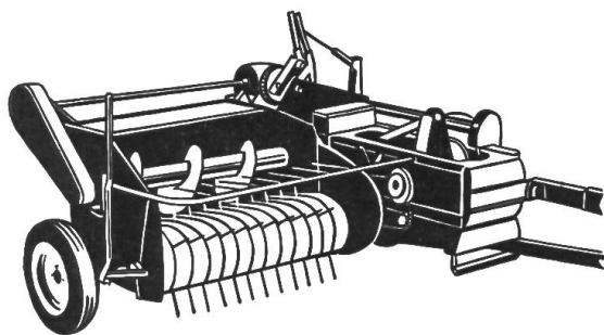
Presse à forte densité 214 B/D pour le foin et la paille. Largeur de ramassage 1,60 m. Rendement horaire: paille 7 tonnes, foin 9 tonnes.
