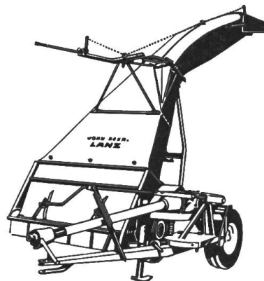
Récolteuse-hacheuse à fléaux FL 110 et FL 140 pour une coupe et un ramassage de la récolte très propres. Largeurs de travail: 100 resp. 140 cm.
