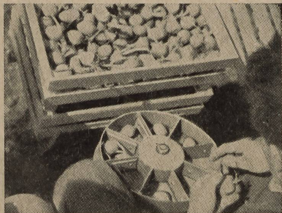
Planteuse semi-automatique avec disque à huit alvéoles pendant la plantation de pommes de terre prégermées.
