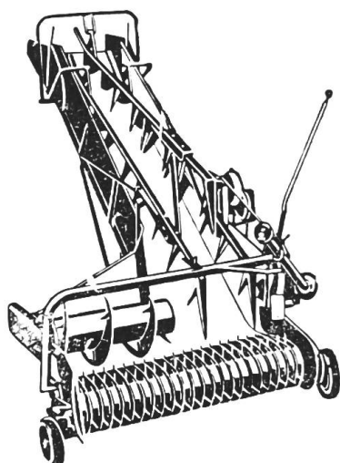
Chargeuse combinée SL 160 avec bande de lancement , pour le chargement du foin, des fourrages verts, du maïs, etc. Largeur de ramassage 1,60 m. Hauteur de charge 3,3 m.
