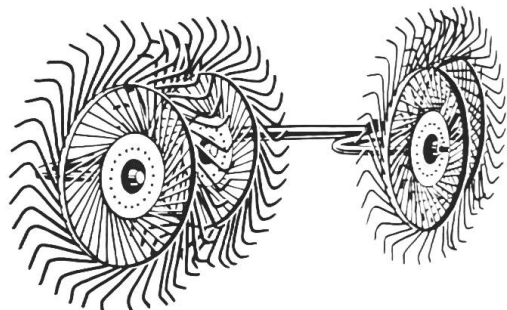
Râteau porté P 140 chenille , attelage 3 points, avec 4 disques souples de 1,40 m, pour l'andainage, le retournement des andains et l'éparpillage.
