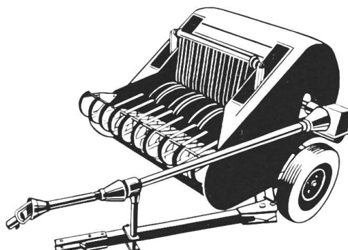
Presse-ramasseuse F 80 pour le pressage et le chargement du foin et de la paille. Largeur de ramassage 1,40 m. Rendement horaire 4 à 8 tonnes.
