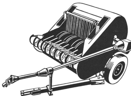
Presse-ramasseuse F 80 pour le pressage et le chargement du foin et de la paille. Largeur de ramassage 1,40 m. Rendement horaire 4 à 8 tonnes.
