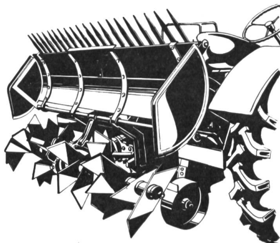
Herses-bêches BUCHER et FAHR attelage 3 points ou relevage à main, 1,40 m et 1,80 m de largeur de travail
