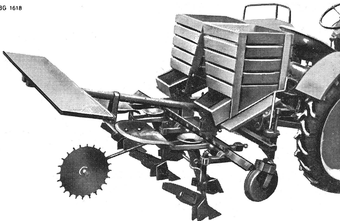
Roue à godets
