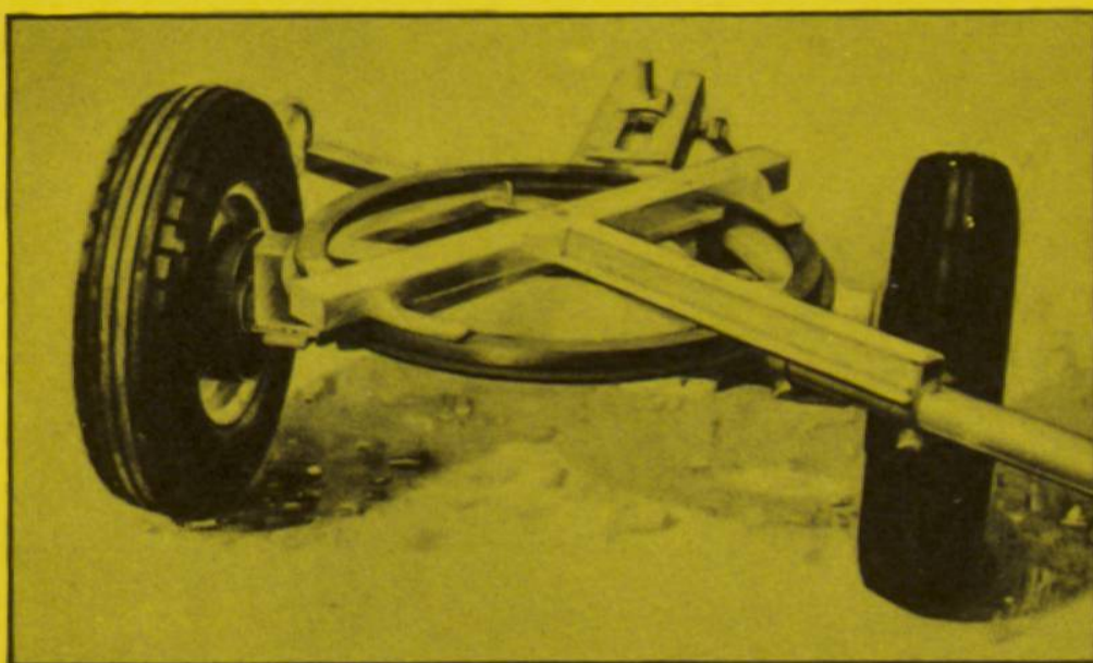
Vorderwagen angeränkt Train avant braqué
