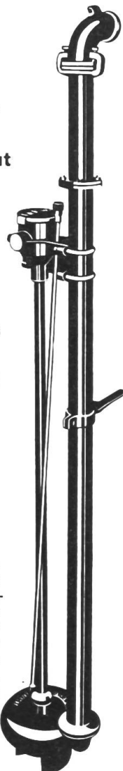
Pompe verticale pour le remplissage du tonneau; s'amorce automatiquement. Engrenages coniques pour commande par transmission ou par moteur électrique accouplé directement. Hauteur de poulie: 2,00 m, 2,25 m, 2,50 m, 2,75 m ou 3,00 m.
