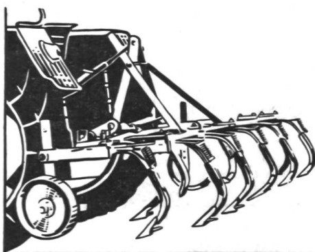
Cultivateur à dents flexibles
