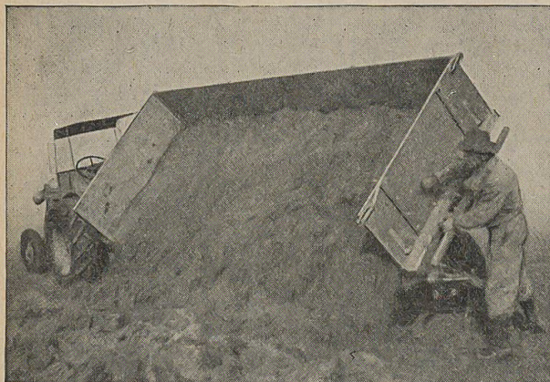
Char à pneus «WM» à pont basculant sur les 2 côtés. Convient tout spécialement pour la traction motorisée.
