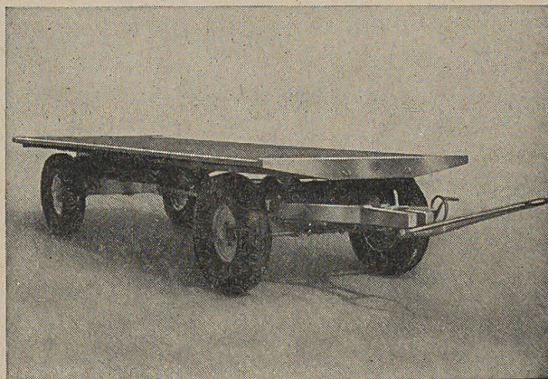
Char à pneus «WM», d'une capacité de charge de 1,5 à 5 tonnes. - Construction entièrement métallique, inoxydable.
