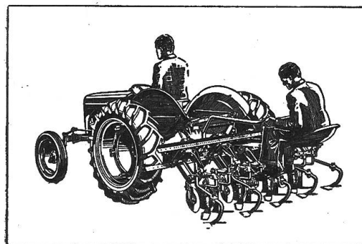
Cultivateur manœuvrable , dents avec disques, couteaux et pattes d'oie réglables facilement, s'emploie avec 1 auxiliaire, pour travail sur 4 lignes (outil spécialement conçu pour culture des betteraves).
