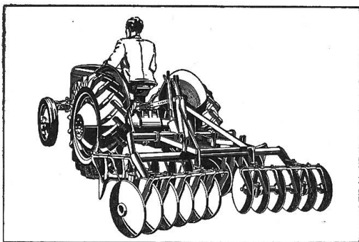
Herse à disques portée attelage aux 3 points. 20 ou 24 disques, 45 cm de diamètre. Largeur de travail 180 cm ou 210 cm. Machine extrêmement robuste et efficace.
