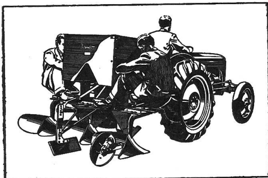
Planteuse de pommes de terre , à 2 rangs, travail pour 2 hommes, en complément avec buttoir à 3 socs Ferguson. Caisse métallique 175 kg. pommes de terre ou 6 caissettes de semence germante.
