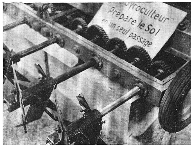
13 Fraise de labour dont les corps travaillent perpendiculairement à la direction d'avancement.
