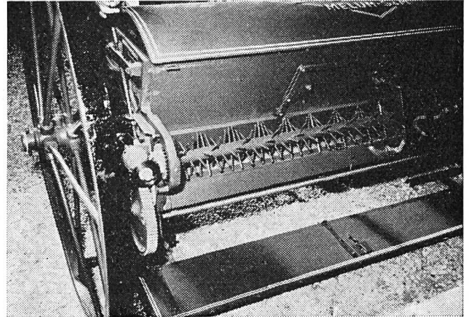
11 Epandeur d'engrais Dumaine à fond mouvant et rouleau épandeur à broches.
