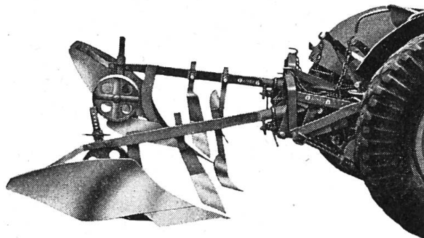
Charrue alternative Althaus, modèle «Dominus»
