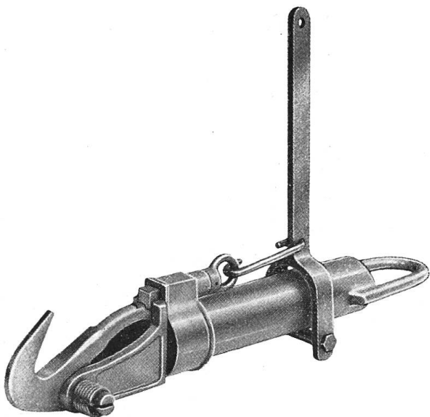
Décrochage automatique Althaus
