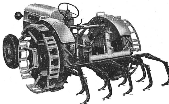
Roues d'adhérence Meili et cultivateur
