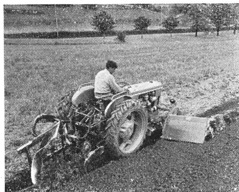
Herse rotative portée Vevey à montage latéral
