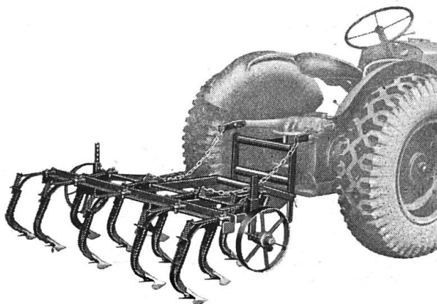
Cadre Althaus pour fixation en 3 points, avec cultivateur
