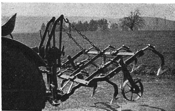
Cultivateur Fenner, Itschnach/ZH
