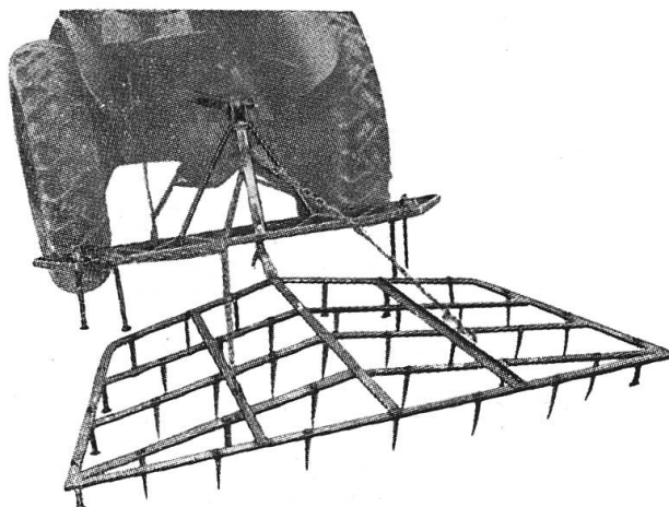
Herse à champs Erismann adaptée à cadre pour fixation en 3 points
