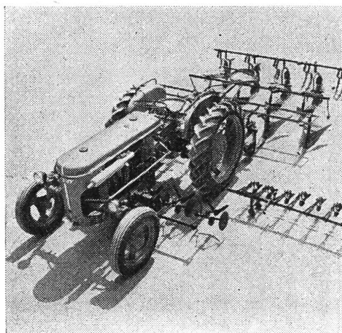
Instruments de sarclage du tracteur Vevey
