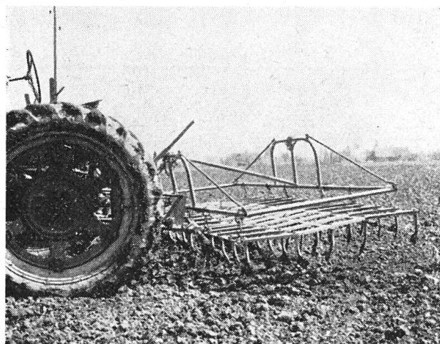
Herse à champs Vogel adaptée à cadre pour fixation en 3 points
