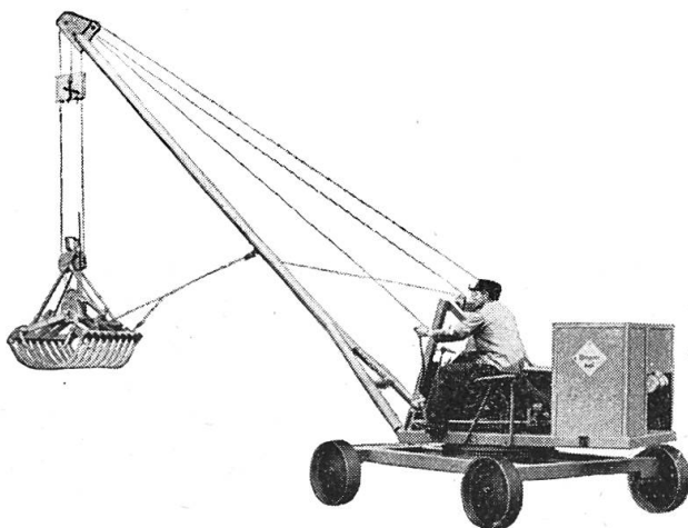
Grue à fumier Mengele
