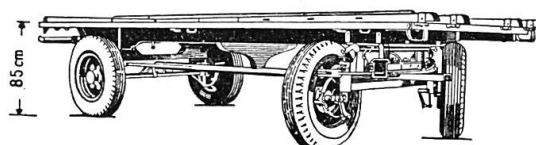
Remorque à deux essieux Neuhaus
