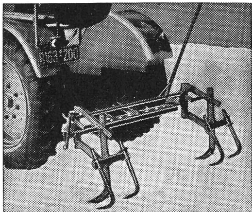
Griffes fouisseuses Degenhart (Griesser, Andelfingen/ZH)
