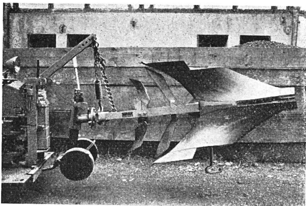
Charrue Ott, modèle 47
