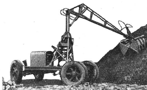
Instrument de chargement Atlas, monté à l'arrière (AIMSA, Genève)
