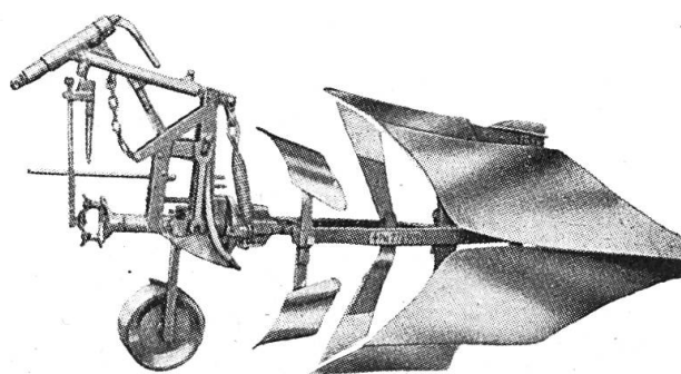
Charrue réversible Erismann pour tracteurs Ferguson et Ford 8 N
