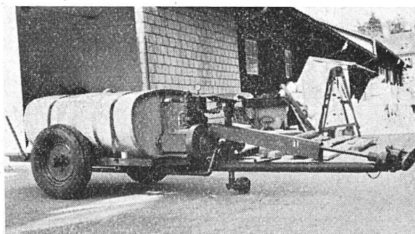
Autre pulvérisateur à haute pression Royal, pour prise de force.
