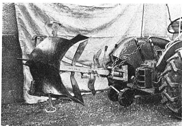
Charrue Ott, modèle 48
