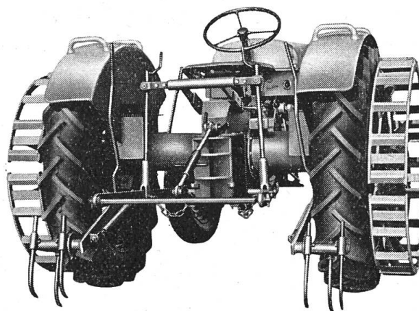
Roues d'adhérence et griffes fousseuses Meili
