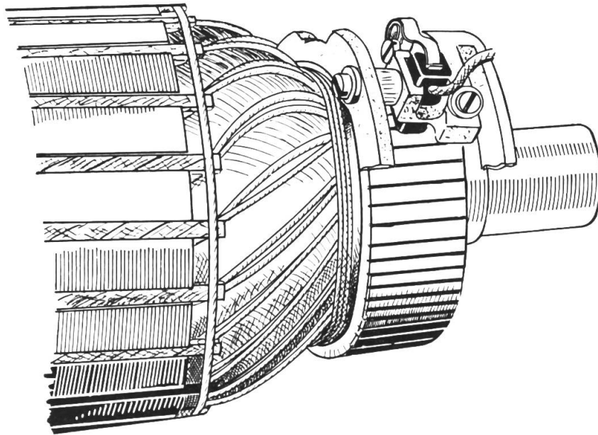
Fig. 141: Vue de détail d'un balai (charbon). Le charbon est légèrement appliqué sur le collecteur par un ressort. L'autre extrémité du carbon est reliée au fil de cuivre qui conduit le courant aux consommateurs (batterie, bobine d'allumage, phares).
