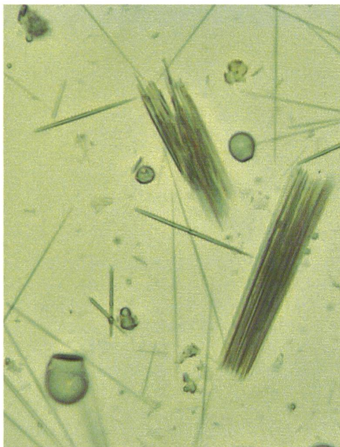
Abb. 3 Gebündelte Raphiden
