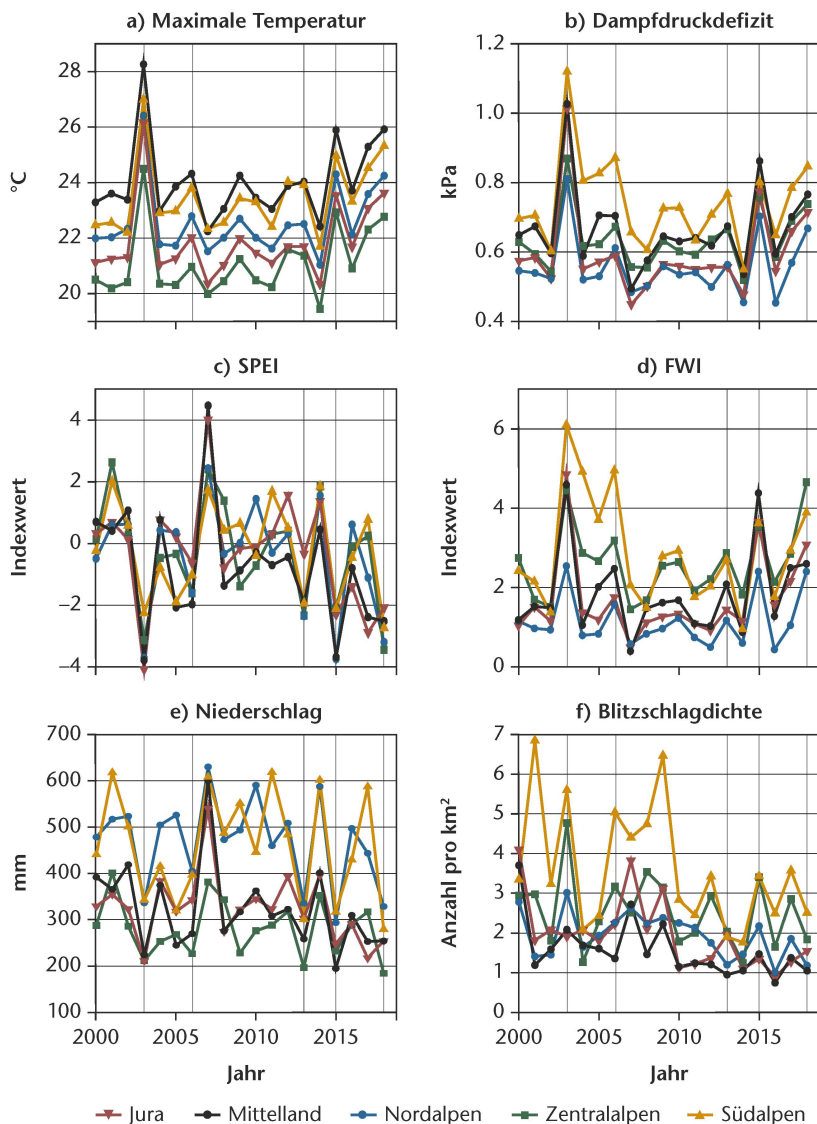
Abb 5 Ausgewählte Meteoroparameter und abgeleitete Indizes im Hochsommer (Juni, Juli, August) der Jahre 2000 bis 2018 in den biogeografischen Regionen. a) mittlere maximale Temperatur, b) Dampfdruckdefizit, c) SPEI-1 Monat (monatlicher Standardized Precipitation-Evapotranspiration Index), d) mittlerer FWI (Canadian Fire Weather Index), e) Gesamtniederschlag und f) Blitzschlagdichte. Die Angaben widerspiegeln den Mittelwert der pro Region genutzten Wetterstationen. In den Abbildungen sind die Blitzschlagbrandjahre 2003, 2006, 2013, 2015 und 2018 mit vertikalen Strichen markiert.
