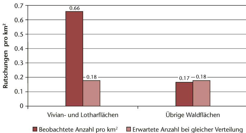
Abb 6 Dichte von flachgründigen Rutschungen in Windurfflächen (Vivian und Lothar, links) und im übrigen Wald (rechts), verglichen mit dem Erwartungswert der Rutschungsdichte über alle Waldflächen (innerhalb und ausserhalb von Windurfflächen). Anzahl Rutschungen: Total = 2208, Vivian = 33, Lothar = 158, übriger Wald = 2017.
