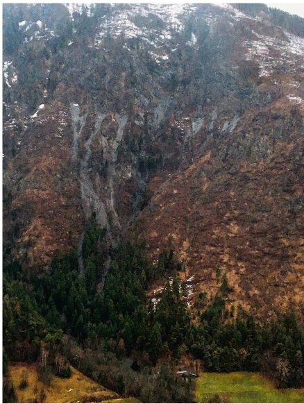
Abb 5 Murgang vom Januar 2018: Entstehungsgebiet (links); prall gefüllter Geschiebesammler (rechts). Im Hintergrund erkennbar ist die potenzielle Ablagerungszone im Wohn- und Industriegebiet Eholz, Visp. Fotos: Alban Brigger
