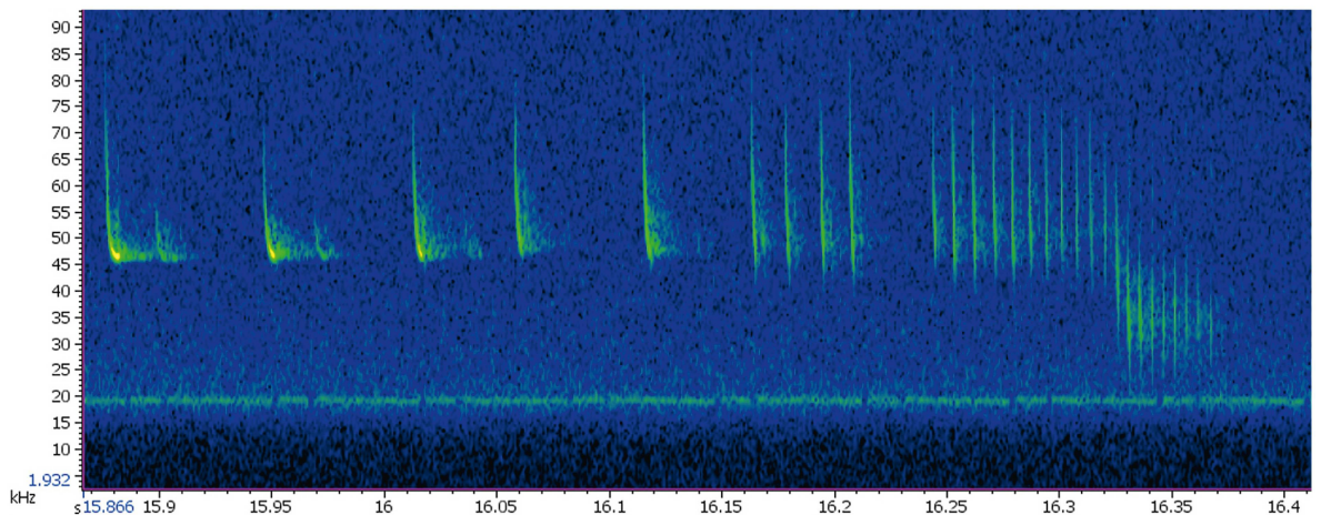
Abb 2 Sonagramm (grafische Darstellung des Frequenzverlaufs [kHz] in der Zeit [s]) mit Ultraschallrufen einer Zwergfledermaus beim Insektenfang.
