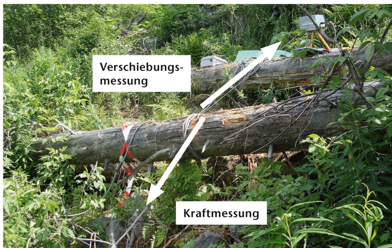
Abb 2 Zugversuche in der Windwurffläche Uaul Cavorgia bei Disentis. Foto: Peter Bebi
