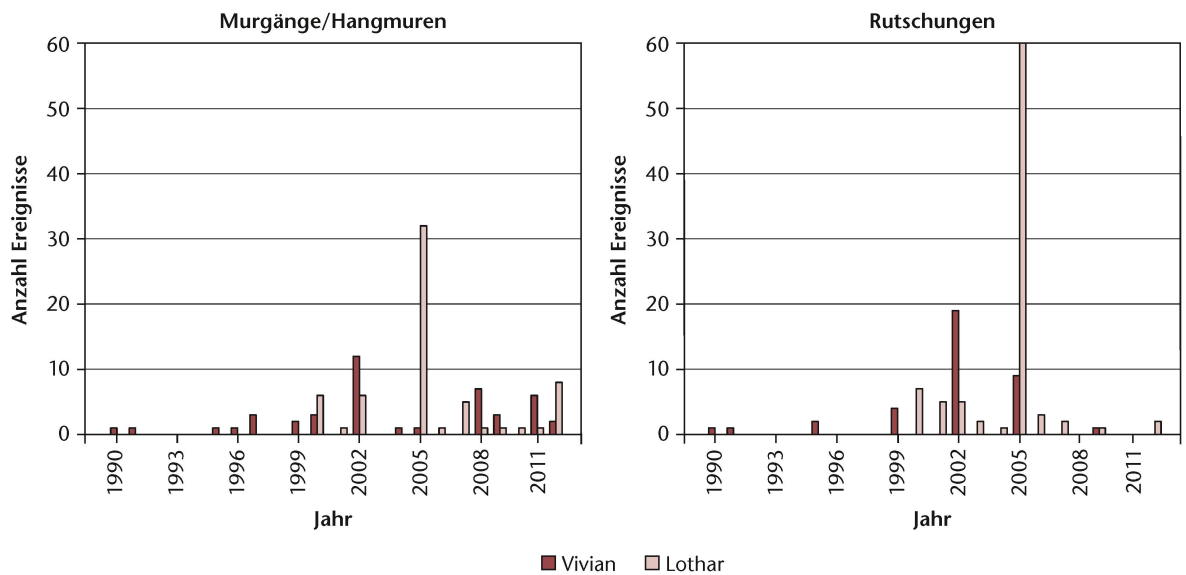
Abb 4 Anzahl Murgänge/Hangmuren und Rutschungen (Anriss- und Transitereignisse) auf Vivian- und Lotharflächen gemäss StorMe-Kataster der Kantone Bern und Graubünden in den Jahren 1990 bis 2013.
