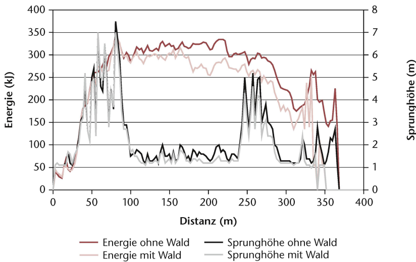
Abb 5 Modellierte maximale Energien und Sprunghöhen der Steine mit und ohne Wald im Profil 7 im Grubenberg (GR) für das 10- bis 30-jährliche Szenario.
