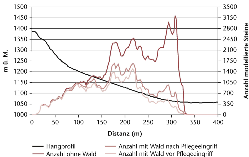
Abb 6 Modellierte Steinschlagaktivität im Profil 7 im Grubenberg (GR) für das 10- bis 30-jährliche Szenario. Bewaldet ist der Abschnitt zwischen 75 m und 320 m ab Ausbruchsstelle.
