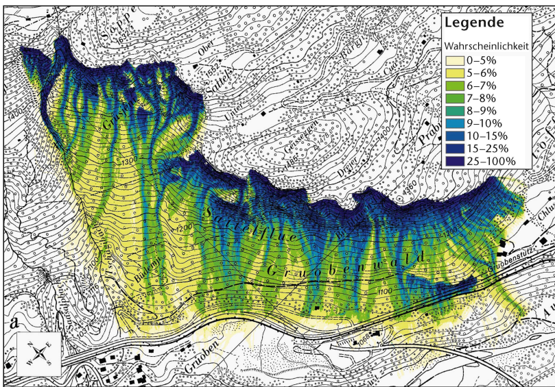
Abb 4 Modellierte Wahrscheinlichkeit für Steinschlagaktivität im Grubenberg (GR) für das 10- bis 30-jährliche Szenario ohne Wald. Je dunkler die Farbe, desto wahrscheinlicher ist das Auftreten von Steinschlag.
