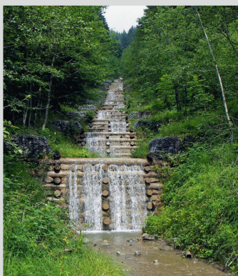
Bachverbau mit Holzsperrn in den Gamser Wildbächen (St. Gallen).
