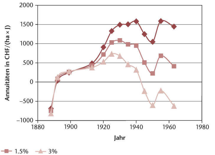
Abb 6 Annuitäten von 1869 bis zum Jahr x (links) und Annuitäten für aufeinanderfolgende Perioden (rechts) für den gleichförmigen Bestand in CHF/(ha x I). Bestandesbegründung 1869 = Jahr 0, Bestandesbegründungs- und Pflegekosten in den ersten 15 Jahren CHF 10 000.-, Zinssatz 0%, 1.5% und 3%.
