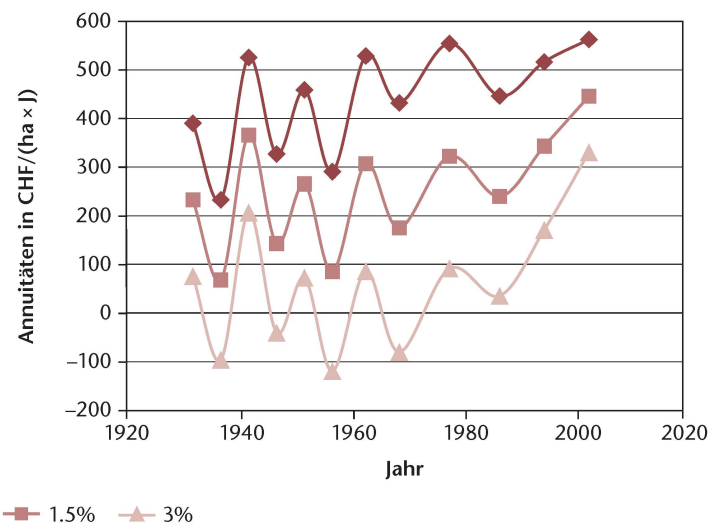
Abb 7 Annuitäten von 1928 bis zum Jahr x (links) und Annuitäten für aufeinanderfolgende Perioden (rechts) für den Plenterbestand in CHF/(ha x I). Erstaufnahme 1928, Zinssatz 0%, 1.5% und 3%.
