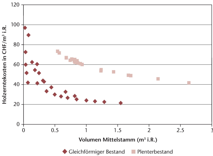
Abb 5 Mit HeProMo (Frutig et al 2009) berechnete und in den beiden Beständen verwendete Holzertekosten.
