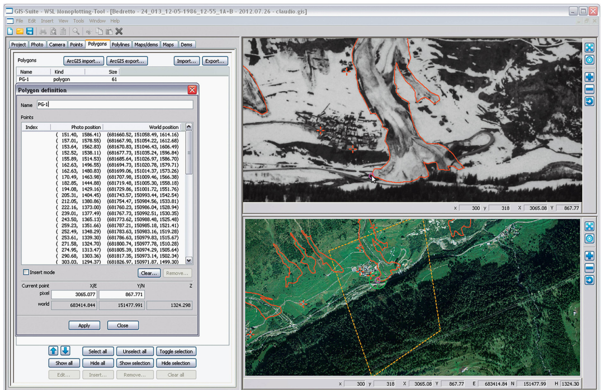
Abb 1 Das Hauptfenster des WSL-Monoplotting-Tools. Rechts oben das Fenster für die Visualisierung und die Navigation auf dem Bild; unten rechts das Fenster für die Visualisierung und die Navigation auf dem Orthofoto (oder auf Landeskarten). Links das Fenster zur Eingabe und Verwaltung der Basisdaten, wobei derzeit das Fenster zur Definition der Polygone aktiviert ist. Wenn das System kalibriert ist, sind beide Bilder georeferenziert, womit sich beide Mauszeiger synchron bewegen. Gleichzeitig werden in der Zeile am unteren Rand der Fenster die entsprechenden Pixel- (Bild oben) und Landeskoordinaten (Bild unten) angegeben. Das gelbe Viereck auf dem Orthofoto grenzt das oben sichtbare Gebiet ab.
