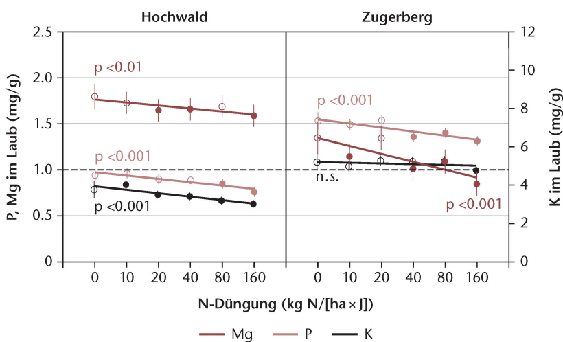
Abb 4 Konzentrationen von P, K und Mg im Buchenlaub in einem N-Düngungsversuch auf Kalk (links) und auf saurem Boden (rechts). Der Grenzwert für Normalversorgung nach Stefan et al (1997) ist als gestrichelte Linie eingezeichnet. Gefüllte Punkte: Unterschied zur Kontrolle signifikant. Aus: Flückiger & Braun (2011).
