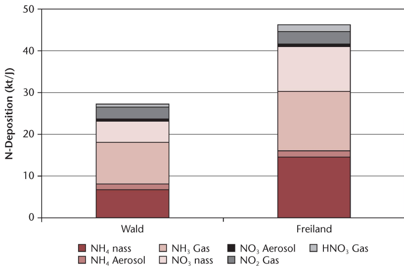
Abb 4 Zusammensetzung der N-Deposition in der Schweiz im Jahr 2007 im Wald (11 382 km 2 ) und im Freiland (29 761 km 2 ; Meteotest 2010).
