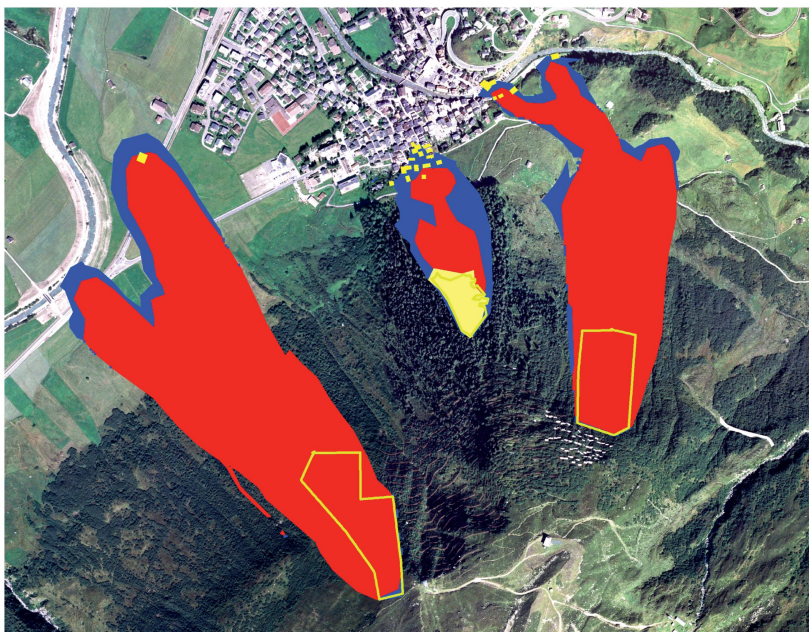
Abb 1 Berechnete Lawinenauslaufzonen für ein 300-jähriges Lawinenereignis in der Gemeinde Andermatt. Rot und blau: rote und blaue Lawinengefahrenzonen; gelbe Fläche: fiktive Windwurffläche; gelb gerahmt: potenzielle Lawinenanrissgebiete.
