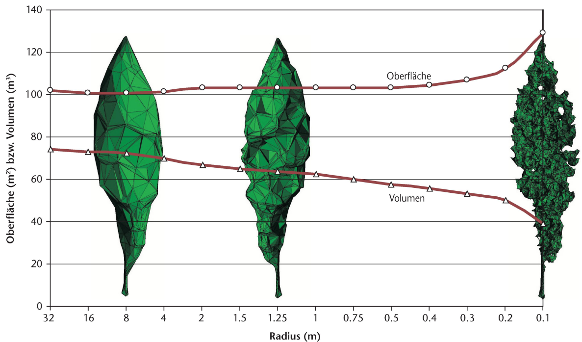
Abb 4 Das Volumen und die Oberfläche verändern sich je nach verwendetem Rekonstruktionsradius \alpha der Alpha-Shapes. Mit kleiner werdendem Radius bleiben mehr Details der Krone erhalten, das Volumen nimmt ab und die Oberfläche nimmt zu.
