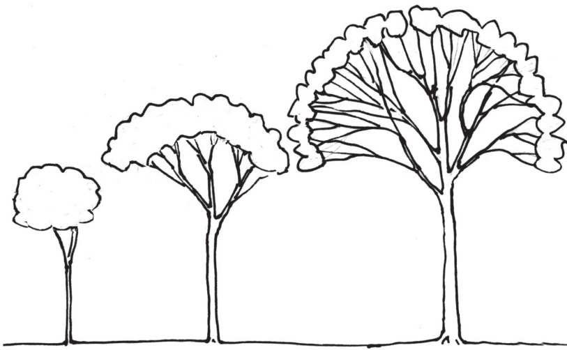
Abb 3 Die unterschiedlichen Prinzipien der Raumfüllung: Beim einen Extrem (links) wird der ganze Kronenraum ausgefüllt, beim anderen (rechts) befinden sich die Blätter nur auf der Aussenhaut der Krone.
