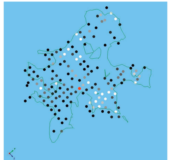
Abb 6 Ein horizontaler Schnitt durch die Dichteverteilung in einer Fichtenkrone bei etwa 50% der Kronenlänge. Die Bereiche über einem Schwellenwert von 10% der Maximaldichte werden durch die Punkte wiedergegeben. Je heller der Punkt, desto dichter ist der zugehörige Raumbereich. Die Grafik beruht nur auf einem einzigen Scan. Die Stammachse ist durch den roten Punkt markiert.
