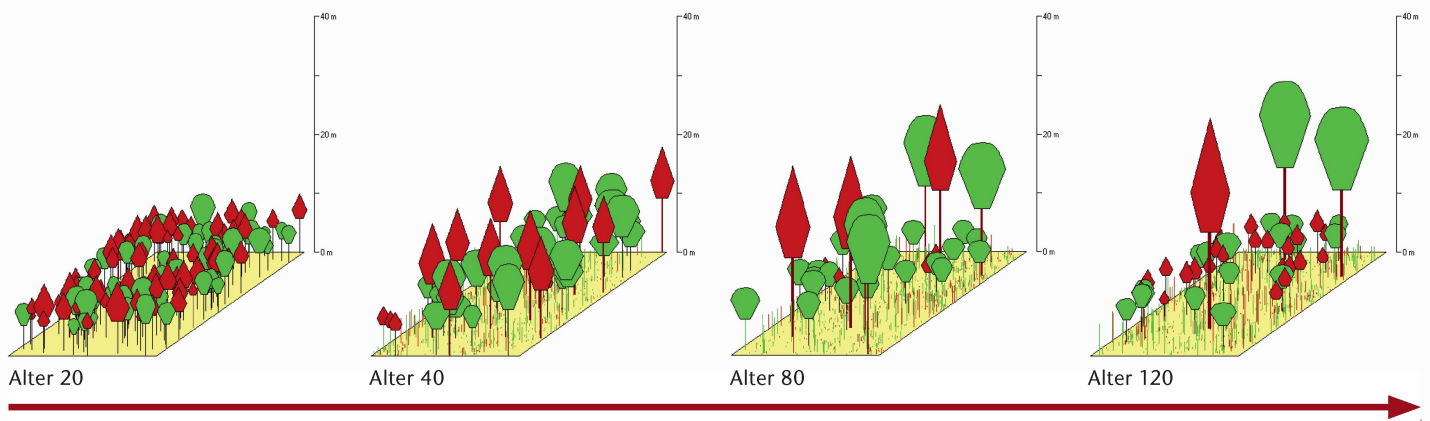
Abb 7 Nutzung von dynamischen Kronenstrukturmodellen für die Simulation und Visualisierung der Baum- und Bestandesdynamik.
