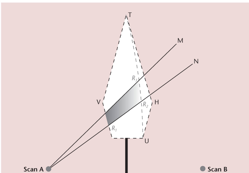
Abb 5 Blattflächenschätzung mittels terrestrischem Laserscanning. Der Baum wird aus zwei gegenüberliegenden Positionen A und B aufgenommen. Die graue Linie zwischen T–U entspricht der Eindringtiefe des Lasers in die Baumkrone beziehungsweise den Punkten, die von Position A aus am weitesten entfernt gemessen wurden. Der Lückenanteil wird nur bis zur Entfernung R_2 bestimmt und ist bei geeigneter Wahl von R_2 eng mit dem Blattflächenindex (LAI) korreliert. Die lokale Blattfläche (LA) wird dann über LA = LAI/(R_2 - R_1) bestimmt.
