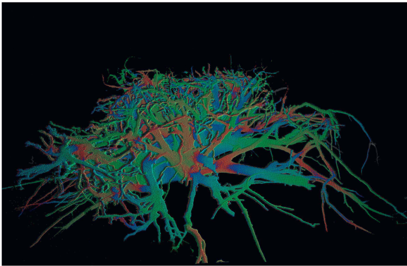
Abb 2 Wurzeln einer 70-jährigen Fichte, erfasst und vermessen mit einem Riegl-LMS-Z360i-Laserscanner in Winkelschritten von 0.12 Grad.
