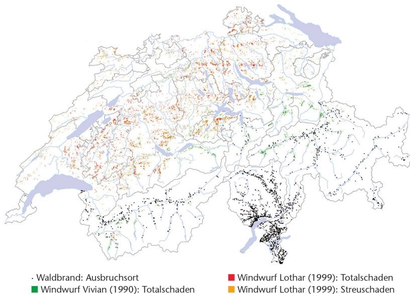
Abb 2 Wind- und Brandstörungen in Schweizer Wäldern: von Vivian (1990) und Lothar (1999) geworfene Waldflächen als Polygone; als schwarze Punkte ohne Flächenangabe die seit 1980 durch Brand zerstörten Wälder in den Kantonen Graubünden, Tessin, Uri und Valais. Vivian-Totalschäden: Mindestfläche 0.2 ha, Restdeckungsgrad maximal 20%; Lothar-Totalschäden: Mindestfläche 1 ha, Restdeckungsgrad maximal 20%; Lothar-Streuschäden: Mindestfläche 1 ha, Restdeckungsgrad Streuschaden zwischen 20% und 60%. Quellen: Vivian- und Lotharinventare: Bafu; Waldbranddatenbank WSL.
