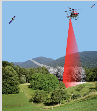
Système de mesure avec LiDAR aéroporté. Montage: Gilles Gachet
