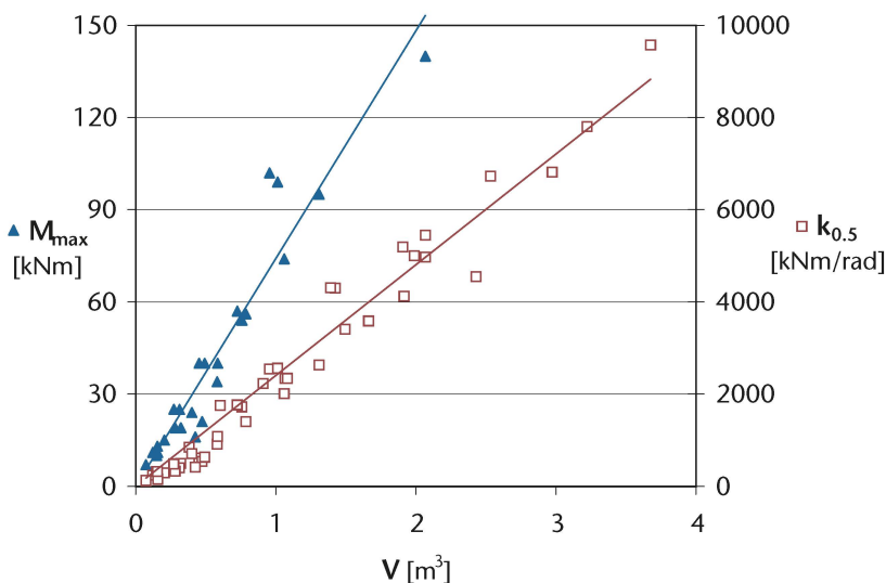
Abb 5 Verankerungseigenschaften. Maximales Verankerungsmoment M_{\max} ▲ und Rotationssteifigkeit k_{0.5} □ in Abhängigkeit des Stammvolumens V : M_{\max} = 74.112 \cdot V ( R^2 = 0.9175 ), k_{0.5} = 2402.2 \cdot V ( R^2 = 0.9628 ).
