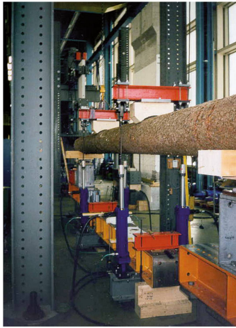
Abb 2 Vier-Punkt-Biegeversuch am frischen Baumstamm.
