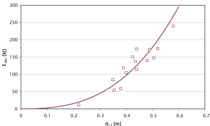
Abb 8 Energieabsorption von Bäumen bei Steinschlag. Maximale Energieabsorption in 1.3 m Höhe E_{abs1.3} □ in Abhängigkeit vom Durchmesser d_{1.3} . E_{abs1.3}=1495.2*d_{1.3}^{3.0335} ( R^2=0.8968 ) [kJ].
