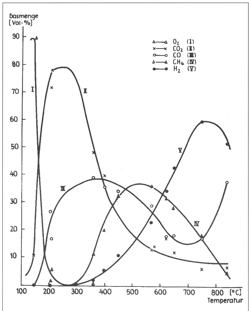
Abbildung 4: Zusammensetzung des Pyrolysegases in Abhängigkeit von der Temperatur.
