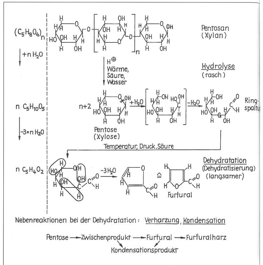
Abbildung 2: Reaktionsschema der Furfuralbildung.
