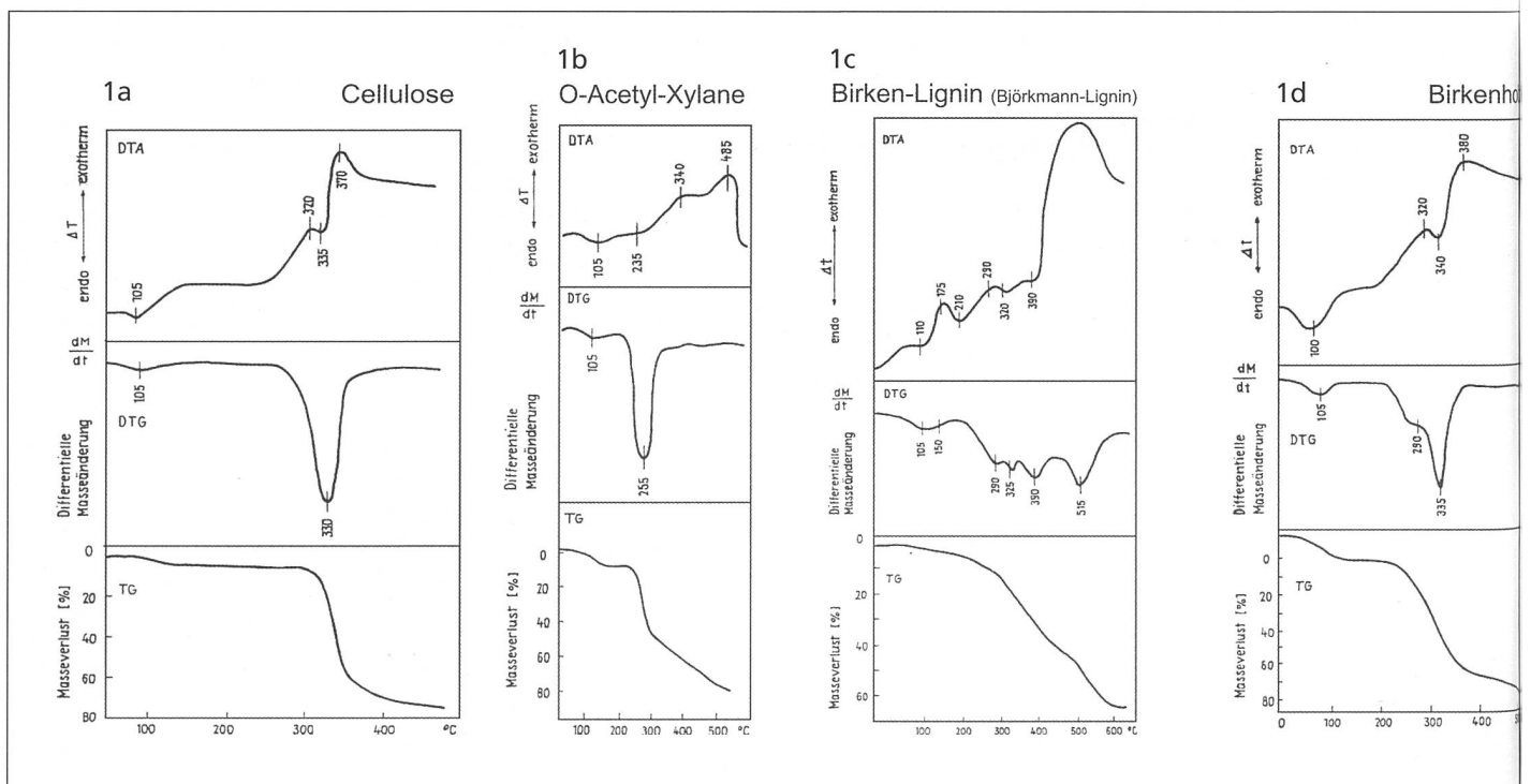
Abbildungen 1a bis 1d: DTA-, DTG- und TG-Kurven verschiedener Holzbestandteile.
