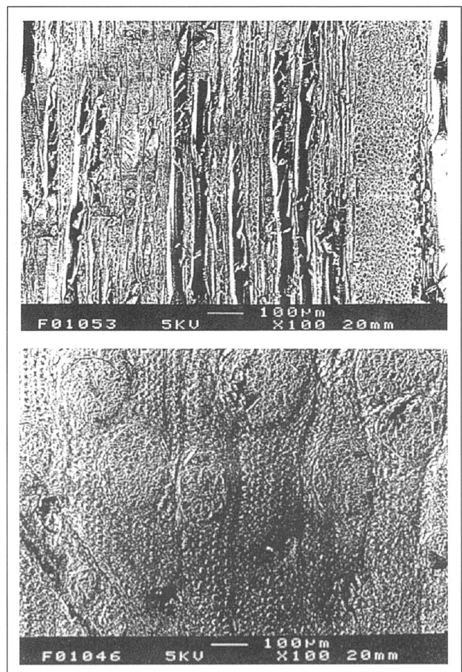
Abbildung 2: REM-Aufnahmen. Einlagerung des mittlerweile ausgehärteten Kunstharzes in die Zelllumen (Fotos: Bauwerk AG).
