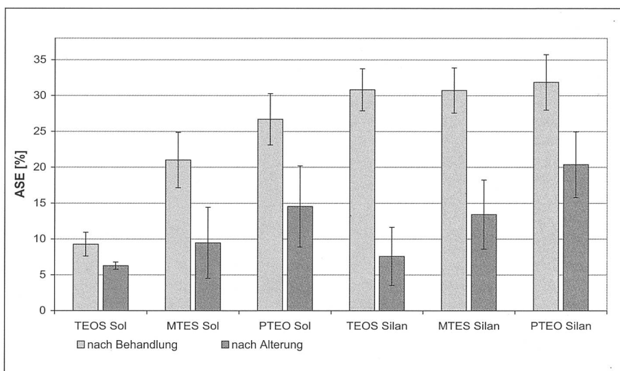
Abbildung 2: Reduzierung der Volumenquellung von Rotbuche durch Behandlung mit Silanen.
