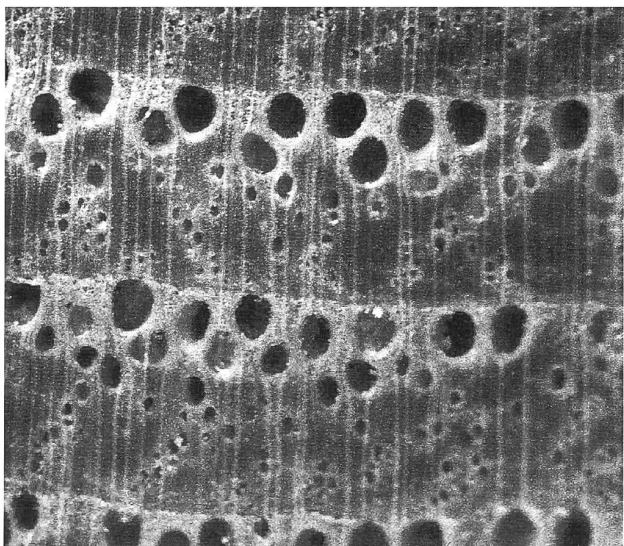
Figura 3: Sezione trasversale del legno di castagno vista al binocolare. Figure 3: Transversal section of chestnut wood (binocular).
