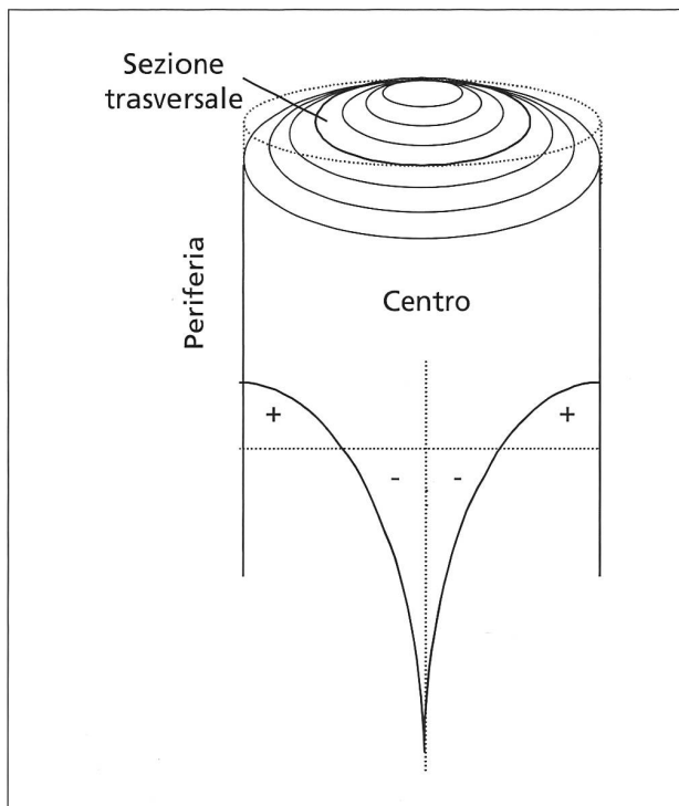
Figura 4: Deformazioni generate dal sezionamento di un tronco. In alto nella figura: cambiamenti dimensionali (esagerati) a seguito della liberazione delle tensioni di accrescimento longitudinali. La parte esterna del cilindro tende a contrarsi mentre quella interna ad espandersi. In basso: distribuzione lungo la sezione di un tronco delle tensioni di accrescimento longitudinali. Le zone di trazione sono segnate con il segno +; quelle di compressione con il segno -. La figura è stata in parte ripresa da KÜBLER (1987).
